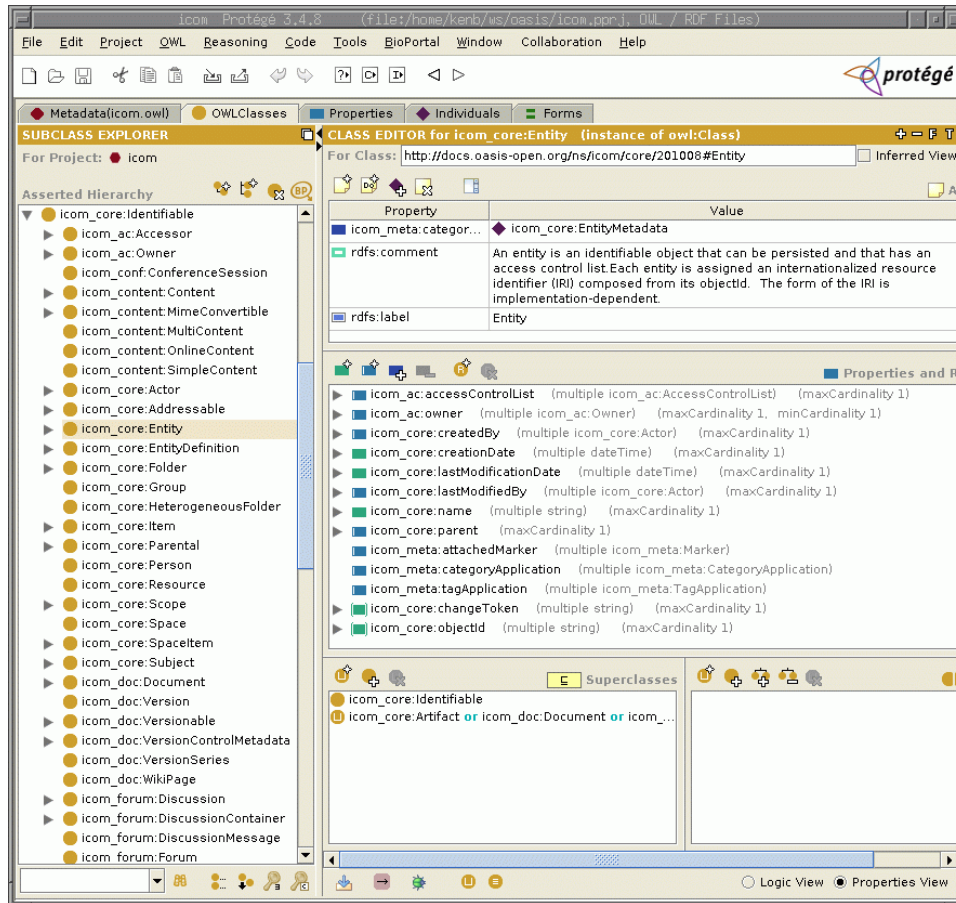
Fig. 5. ICOM Entity Class in Protégé
